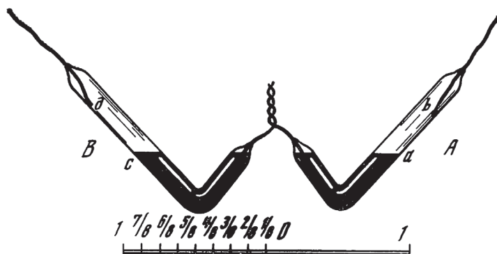
Рис. 29 Ртутный соединительный прибор Б.С.Якоби простейшего типа
