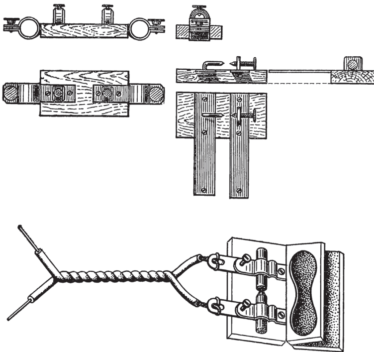
Рис. 26 Электрический минный запал П.Л.Шиллинга а – ранний тип; б – последний тип
