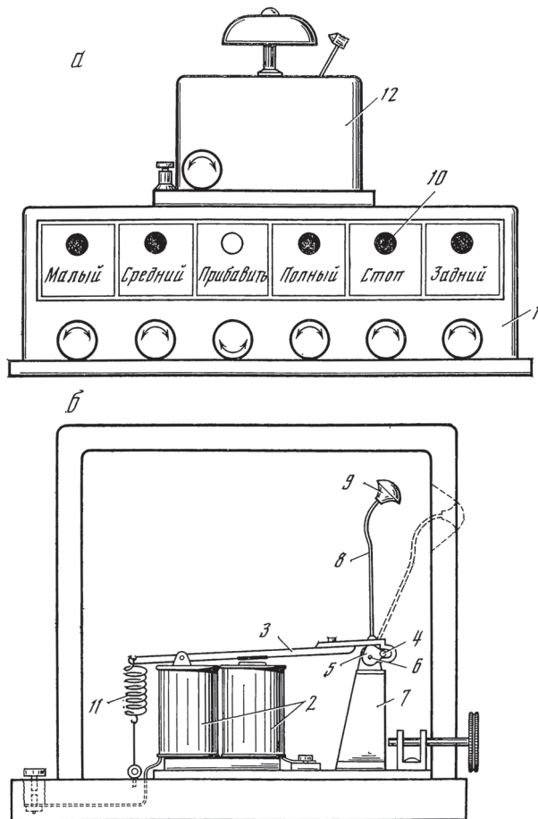
Рис. 25 Корабельный телеграф Б.С.Якоби, установленный в 1855 г. на паровом фрегате «Полкан» для связи между капитаном и машинным отделением: а – внешний вид приемника; б – электромагнитное устройство приемника
