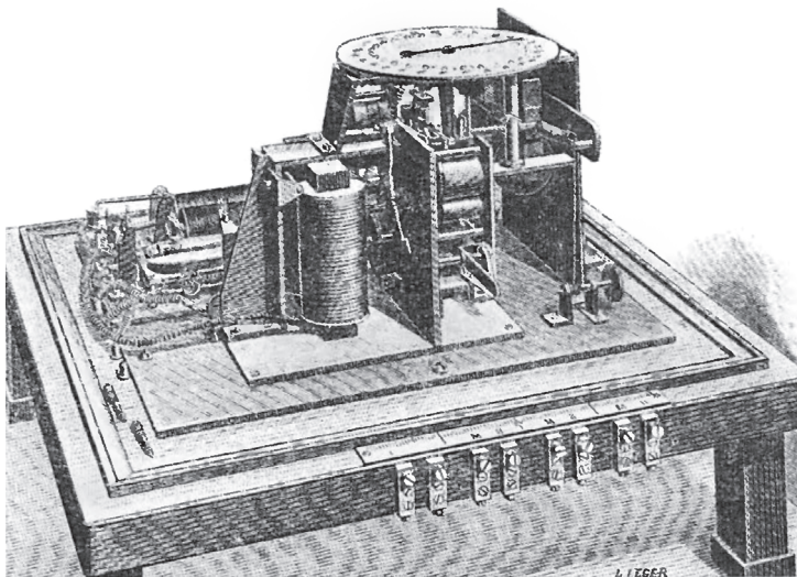
Рис. 24 Буквопечатающий телеграфный аппарат Б.С.Якоби (1850 г.)
