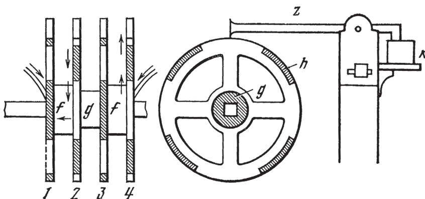
Рис. 2 Коммутатор электродвигателя Б.С.Якоби
