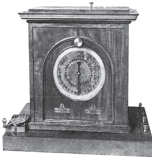
Рис. 21 Стрелочный телеграфный аппарат Б.С.Якоби вертикальной формы со штепсельным передатчиком (1843 г.)
