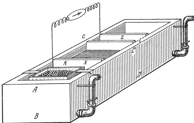
Рис. 10 Одна из сконструированных Б.С.Якоби гальванопластических ванн
