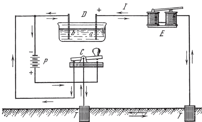
Рис. 18 Схема включения контрбатареи Б.С.Якоби в телеграфную линию
