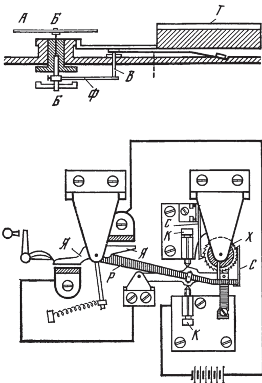
Рис. 23 Принцип действия горизонтального стрелочного телеграфного аппарата
