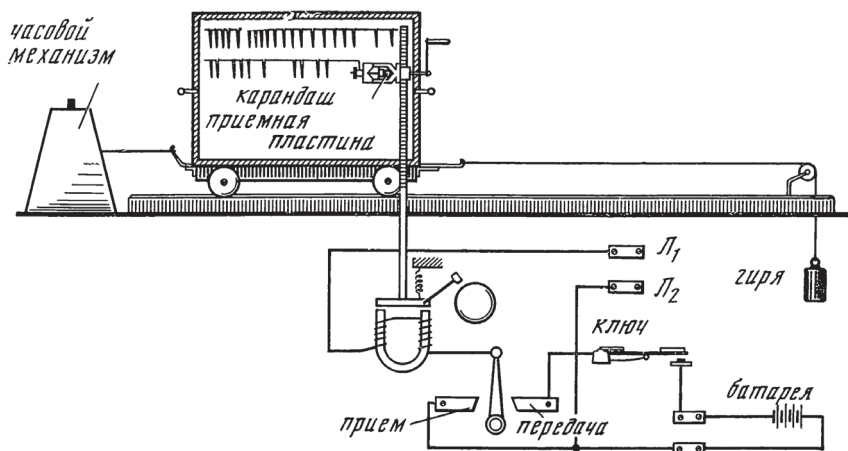
Рис. 17 Принципиальная схема пишущего телеграфного аппарата Б.С.Якоби
