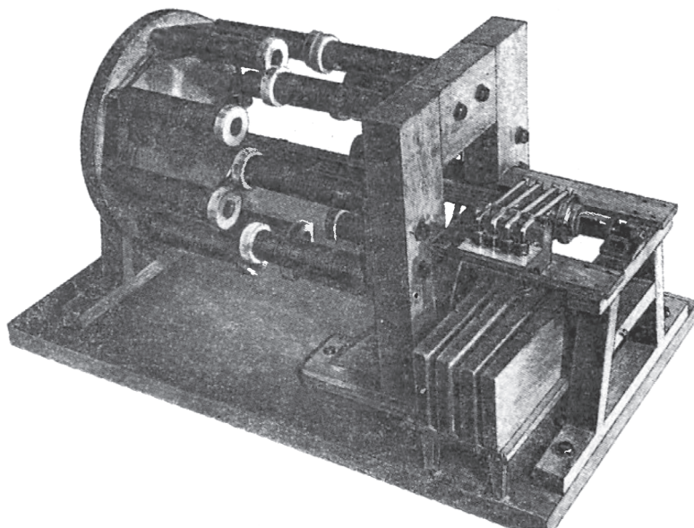
Рис. 1 Электродвигатель Б.С.Якоби конструкции 1834 г.
