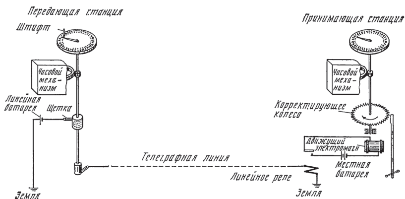
Рис. 20 Принцип действия стрелочных телеграфов Б.С.Якоби
