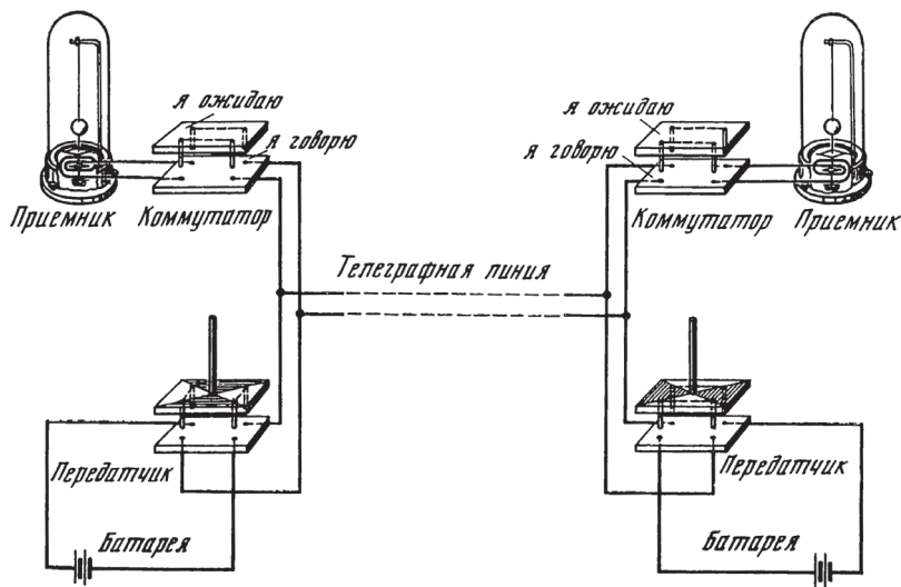
Рис. 11 Принципиальная схема одномультимплекторного телеграфа П.Л.Шиллинга
