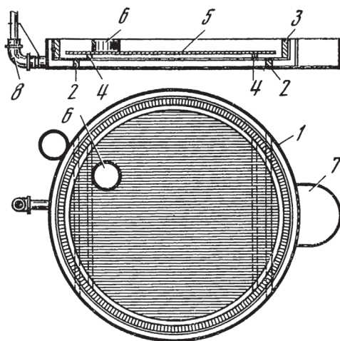
Рис. 6 Гальванический элемент конструкции Б.С.Якоби
