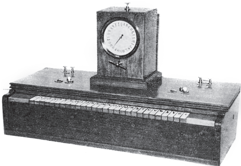
Рис. 22 Стрелочный телеграфный аппарат Б.С.Якоби горизонтальной формы с прямой клавиатурой (1845 г.)
