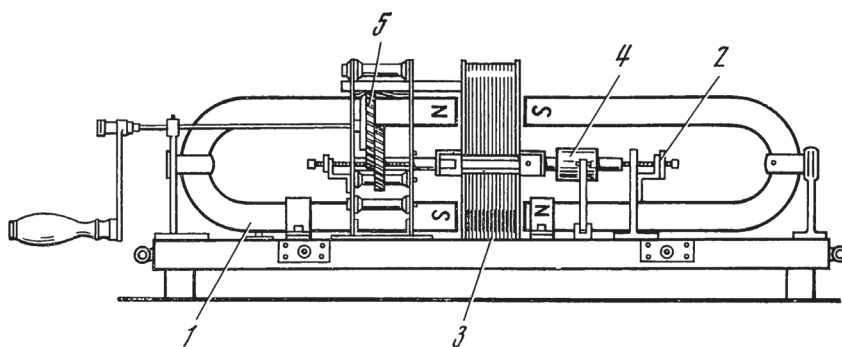
Рис. 31 Магнитоэлектрический генератор Б.С.Якоби
