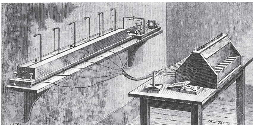
Рис. 12 Шестимультимпликаторный телеграфный аппарат П.Л.Шиллинга в том виде, как он демонстрировался на Парижской электротехнической выставке 1881 г.
