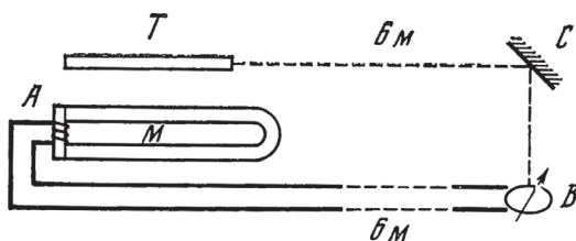
Рис. 7 Схема баллистического метода измерения силы тока, использованная Э.Х. Ленцем и Б.С.Якоби при исследованиях электромагнитов
