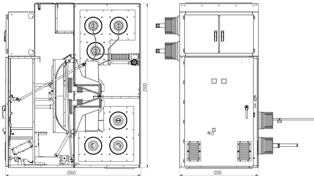
Рис. П2.9 Шкаф КРУ D-40P с НССШ СР
